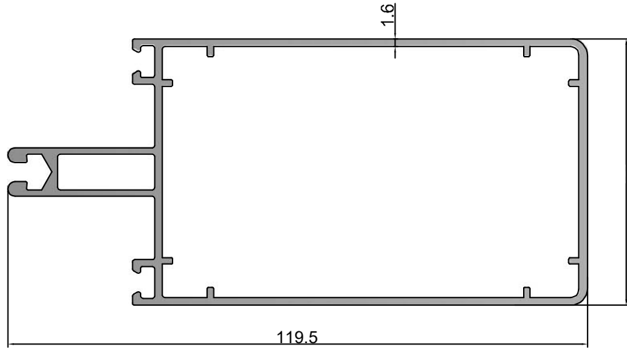
Kod : 4689 Taşıyıcı Profil
