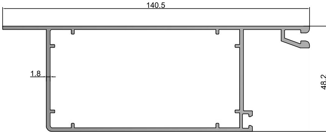
Kod : 4695 Bitim Kapak Profili
