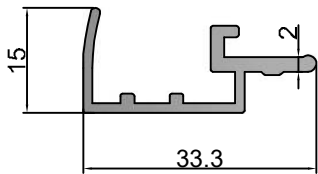
Kod : 4690 Alın Profili Teorik Ağırlık : 0.283 kg/m
