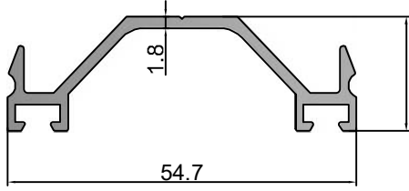
Kod : 4697 Kapak Baskı Profili Teorik Ağırlık : 0.464 Kg/M
