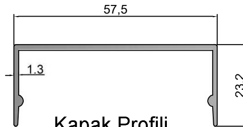
Kapak Profili Kod : 4696
