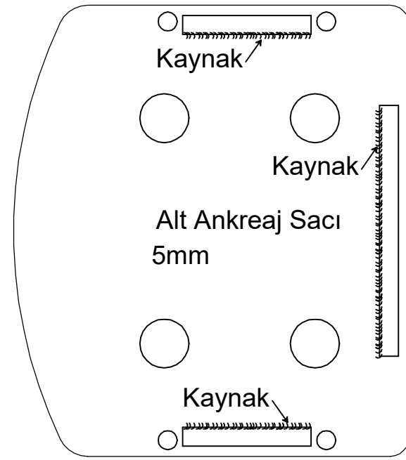
20-700-019 Ankraj 5mm Sac Levha Boyalı
